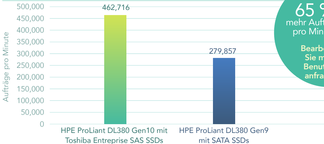
Aufträge pro Minute (höher ist besser)
